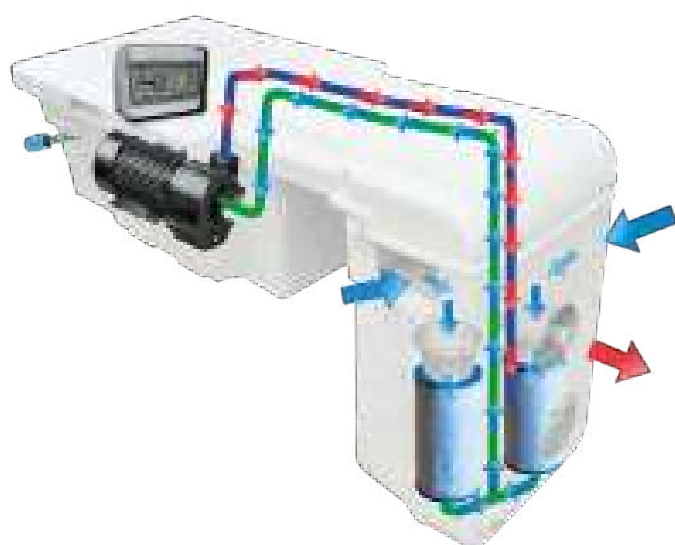
Schéma hydraulique du bloc filtrant (standard hors options)
